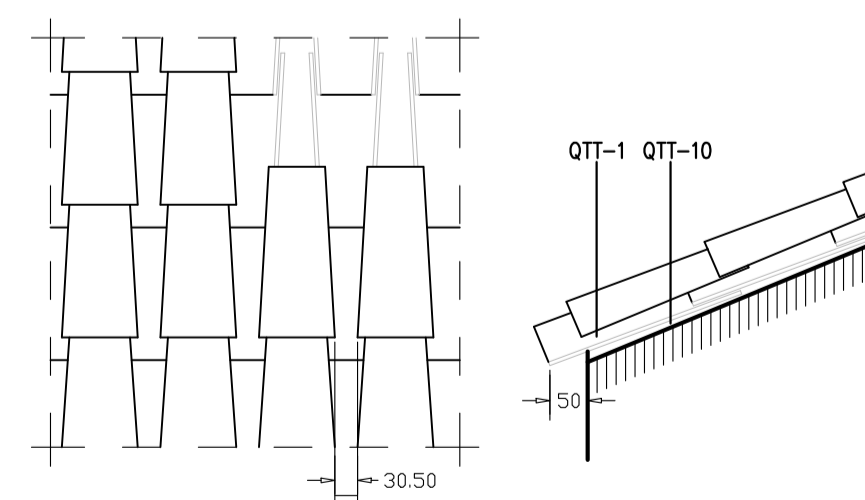
QTT-14 ALERO TEJA CURVA-Tipo
