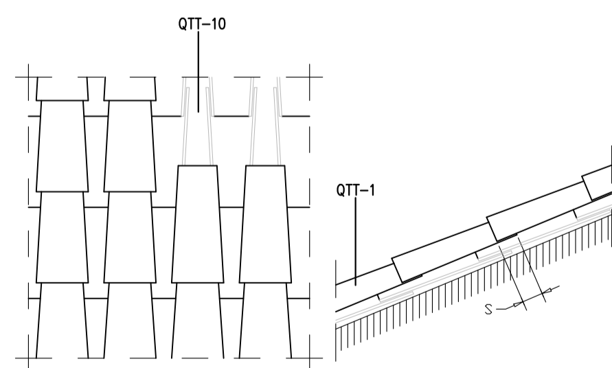
QTT-11 FALDON DE TEJA CURVA-S-Tipo
