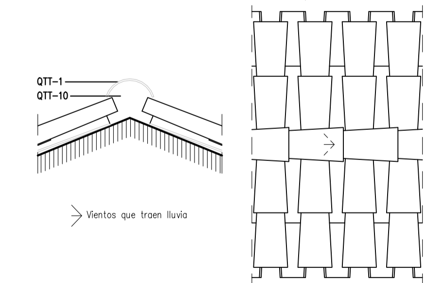
QTT-19 CUMBRERA DE TEJA CURVA-Tipo
